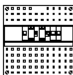
Installatiekast 3x achter 2 aardlekschakelaar 2x 30mA 1-fase
