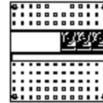
Installatiekast met 3x patroonlastscheiders 16A
