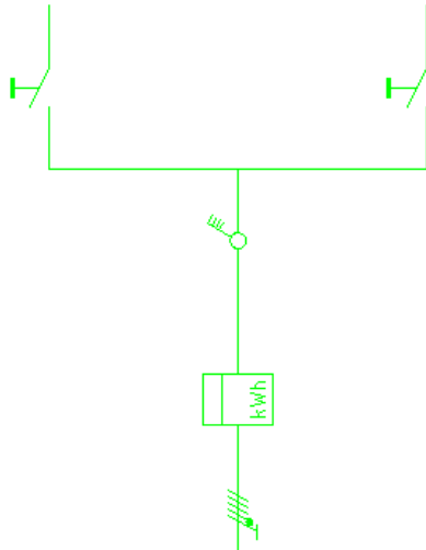
Hoofdschakelaar 4-polig met kWh meter en 1 aardlekautomaat
