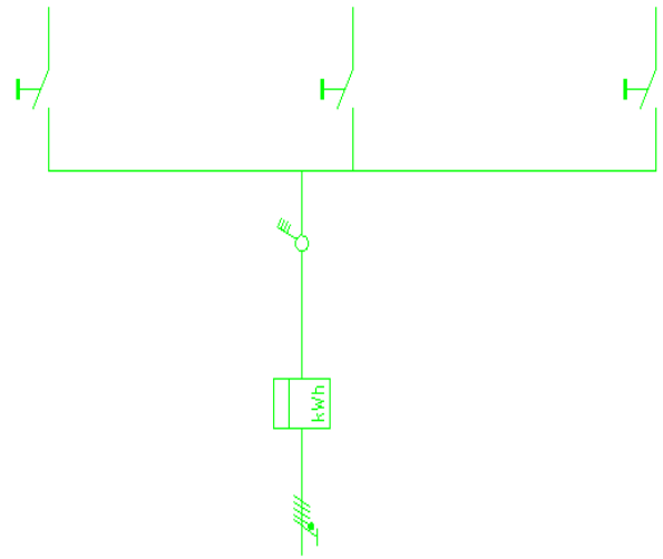
Hoofdschakelaar 4-polig met kWh meter en 3 aardlekautomaten
