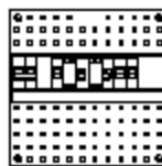
Installatiekast 3x achter 2 aardlekschakelaar 2x 30mA +
