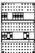
Installatiekast 4x achter 2x 30mA + F + hoofdschakelaar 1-fase
